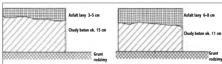
Rzeczywisty układ warstw nawierzchniowych z dwóch odwiertów
