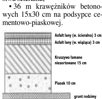
Układ warstw wg. kosztorysu powykonawczego
