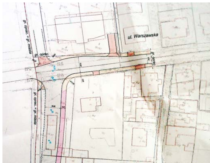
skrzyżowanie Nowoprojektowanej z Warszawską
